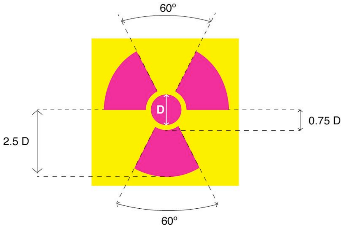
Figura AN1. Señal para indicar presencia de radiaciones ionizantes
